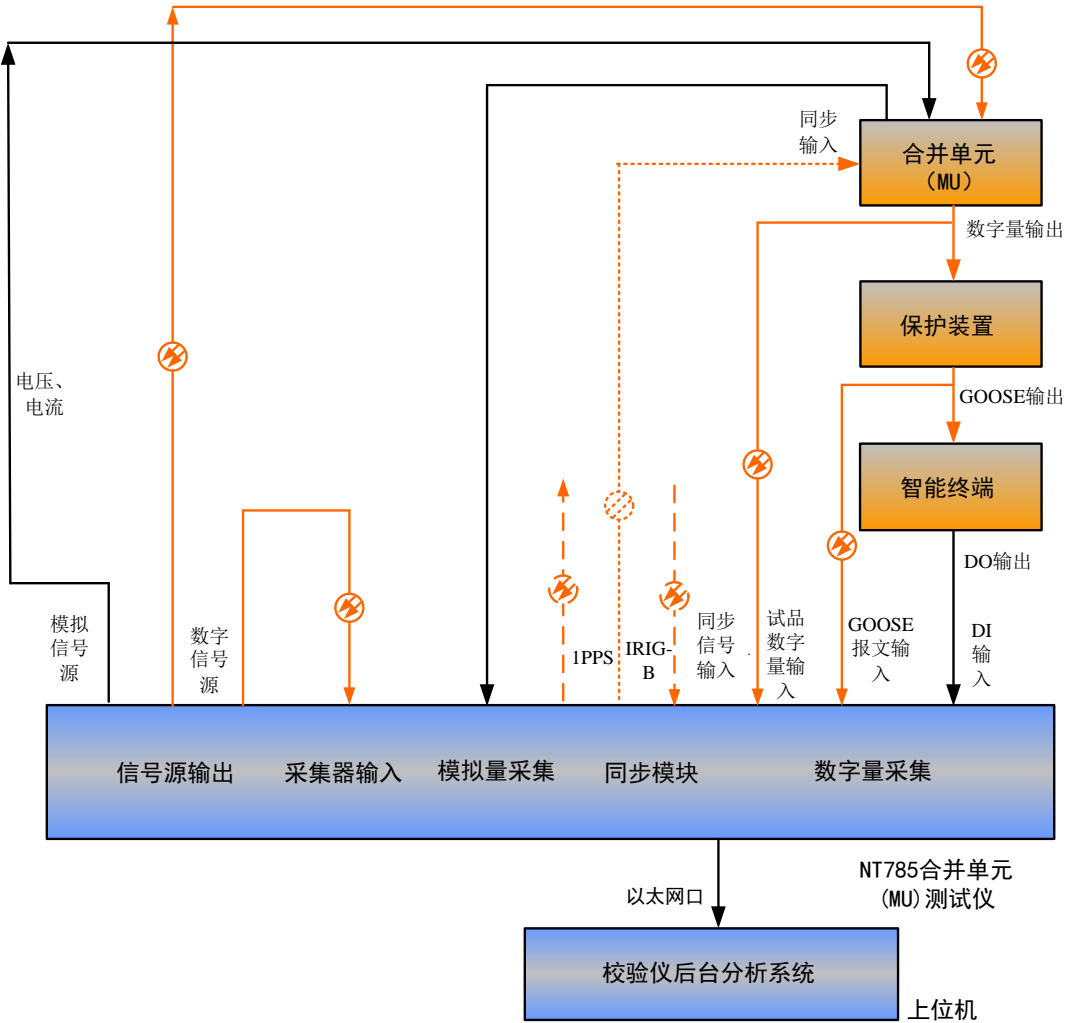
图 1 测试系统结构示意图
