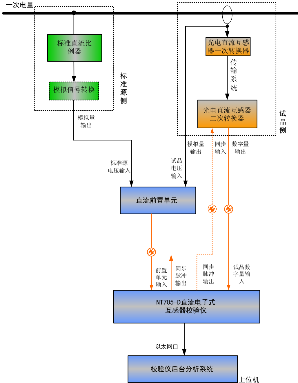
图 1 校验系统结构示意图
