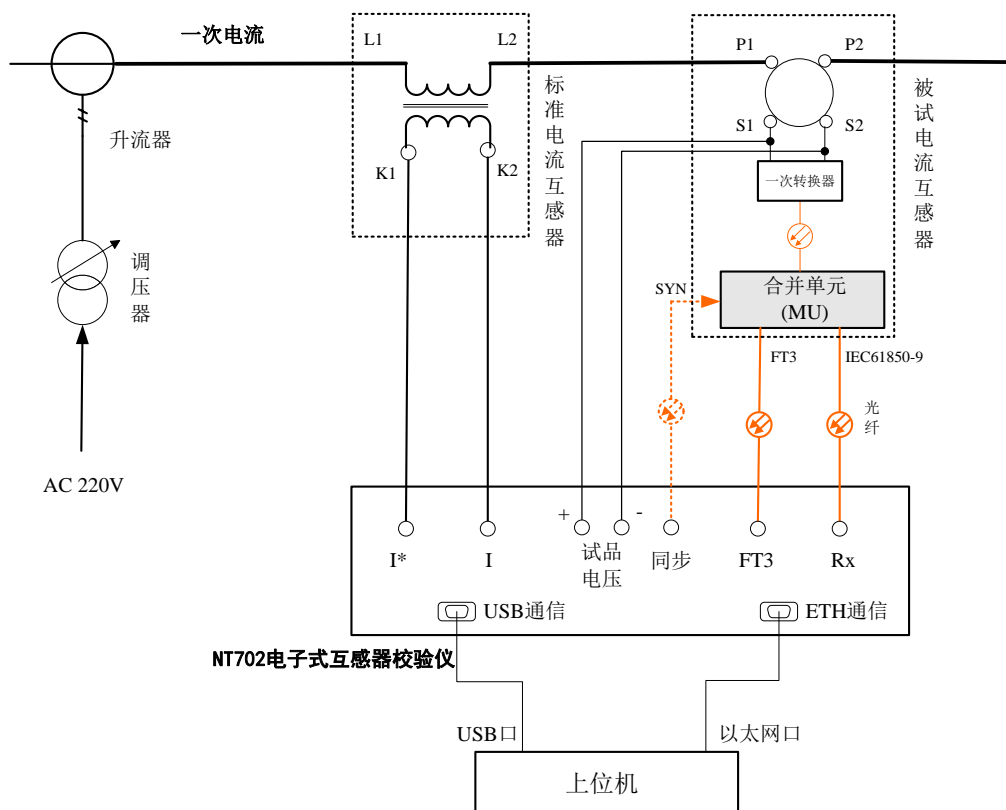
图9 电子式电流互感器试验参考接线
