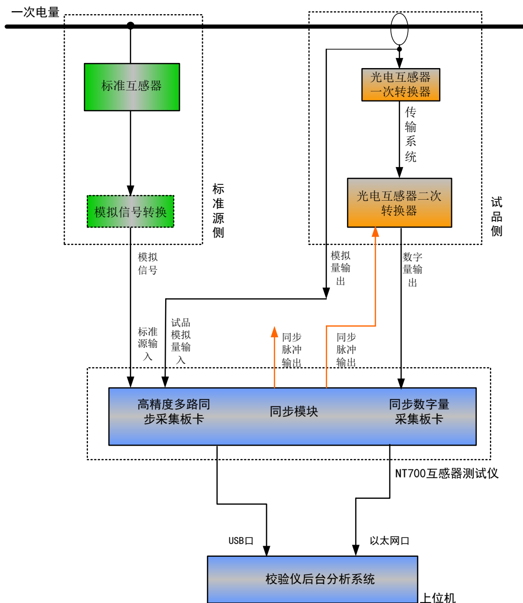
图 1 稳态校验系统结构示意图
