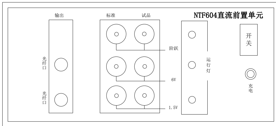
图 4 前置单元面板示意图
