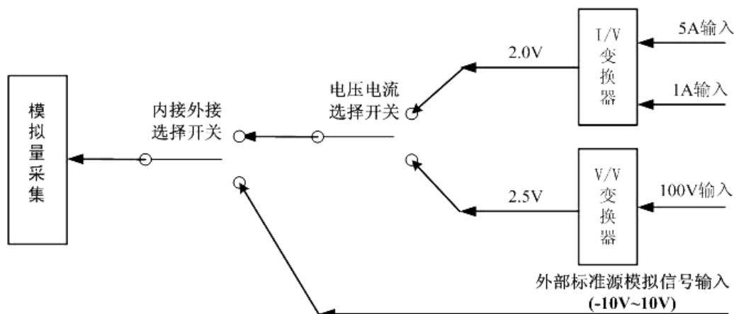
图 7 标准源信号接入方式
