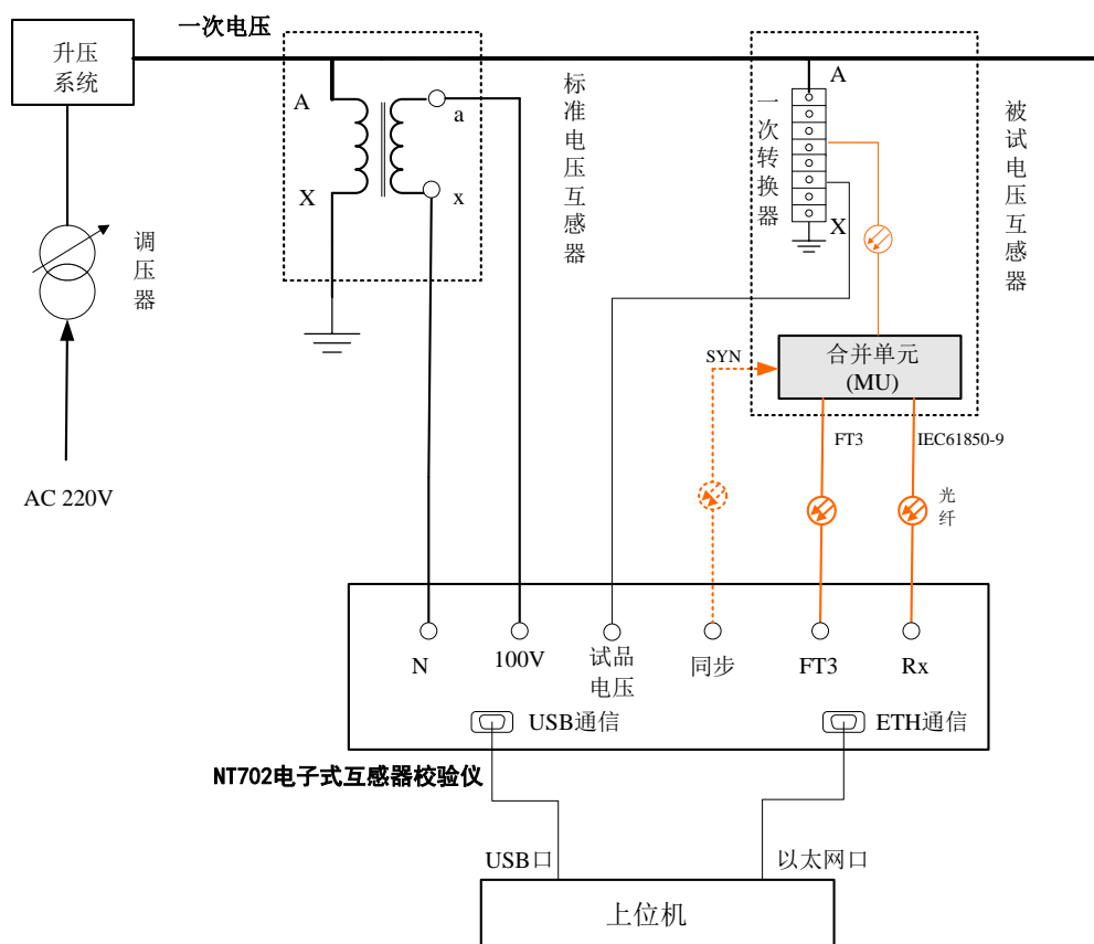
图 10 电子式电压互感器试验参考接线
