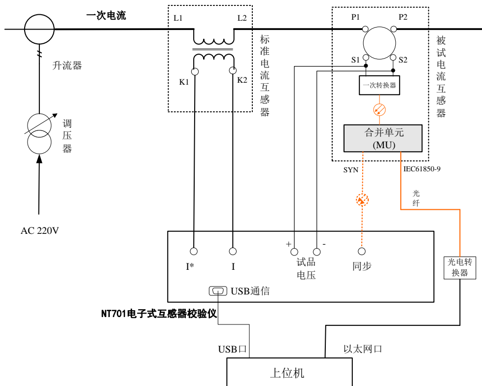
图 13 电子式电流互感器试验参考接线
