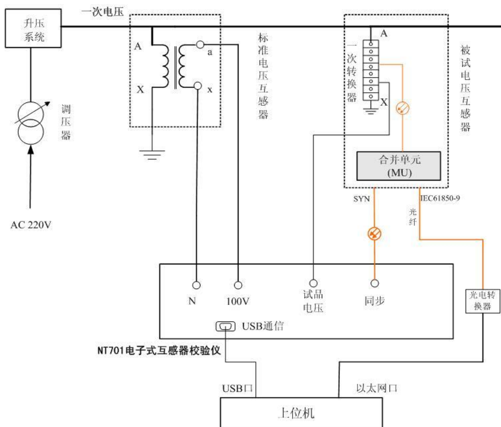
图 14 电子式电压互感器试验参考接线
