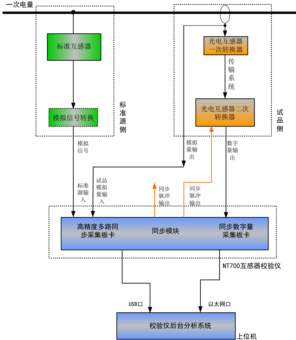
图1 稳态校验系统结构示意图
