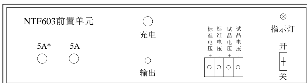
图3 前置单元面板示意图
