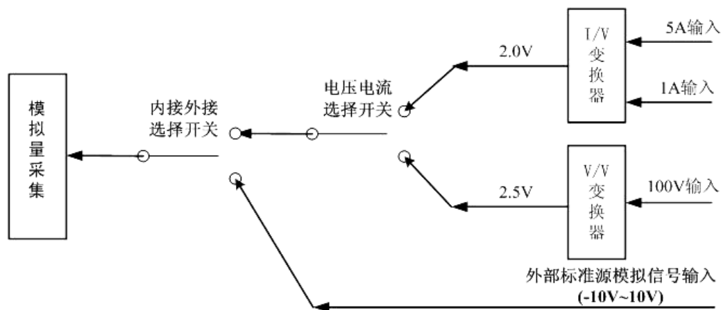
图 12 标准源信号接入方式
