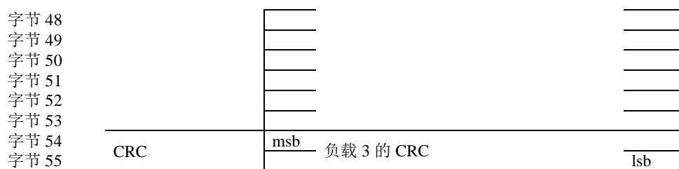
图 2 依据 FT3 的帧格式
