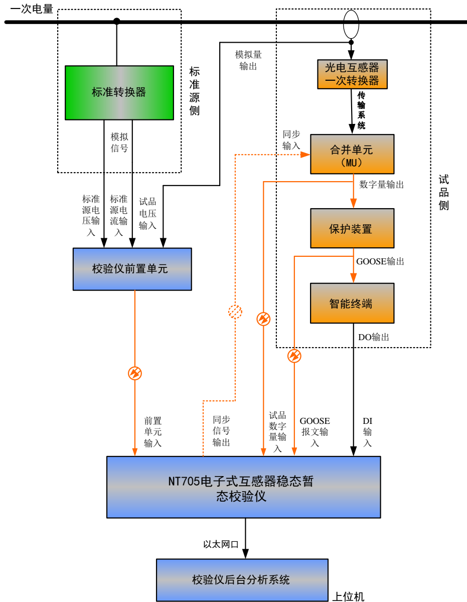
图2 暂态校验系统结构示意图
